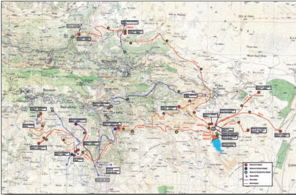
موقع السد وشبكة توزيع المياه على البلدات
